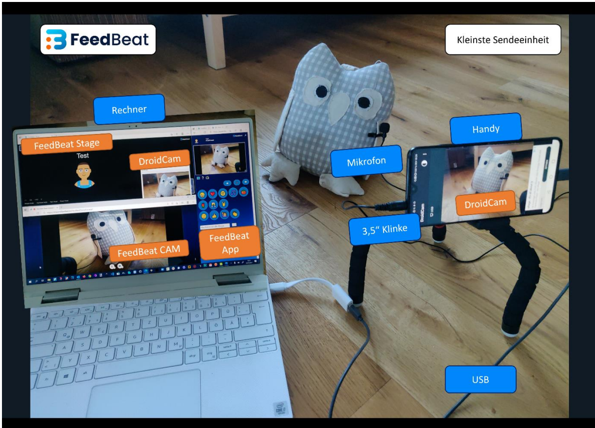
Abbildung 4: Kleinste Sendeeinheit
